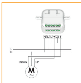
Aansturing van een 230VAC-motor
