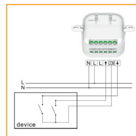
Aansturing van een potentiaalvrij contact
