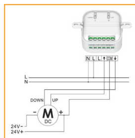
Aansturing van een 24Vdc-motor
