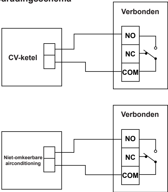
Bedradingsschema
