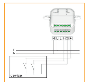
Control de un contacto seco
