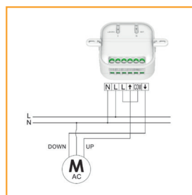
Control de un motor de 230 V ca
