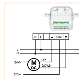
Control de un motor de 24 V cc
