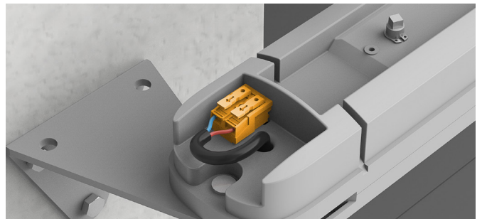
KLEMMLEISTE OHNE WERKZEUG
