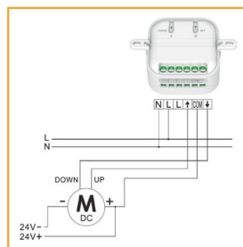
Steuerung eines 24 V-Gleichstrommotors
