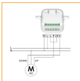
Steuerung eines 230 V-Wechselstrommotors
