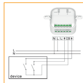
Steuerung eines potentialfreien Kontakts
